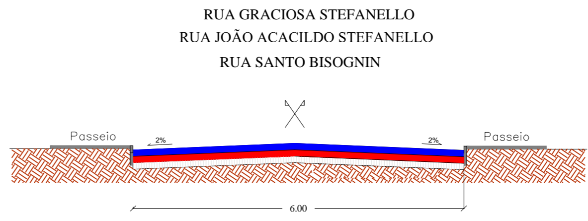
SEÇÃO TRANSVERSAL - TIPO
