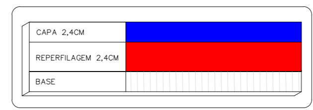
SEÇÃO TRANSVERSAL - TIPO
